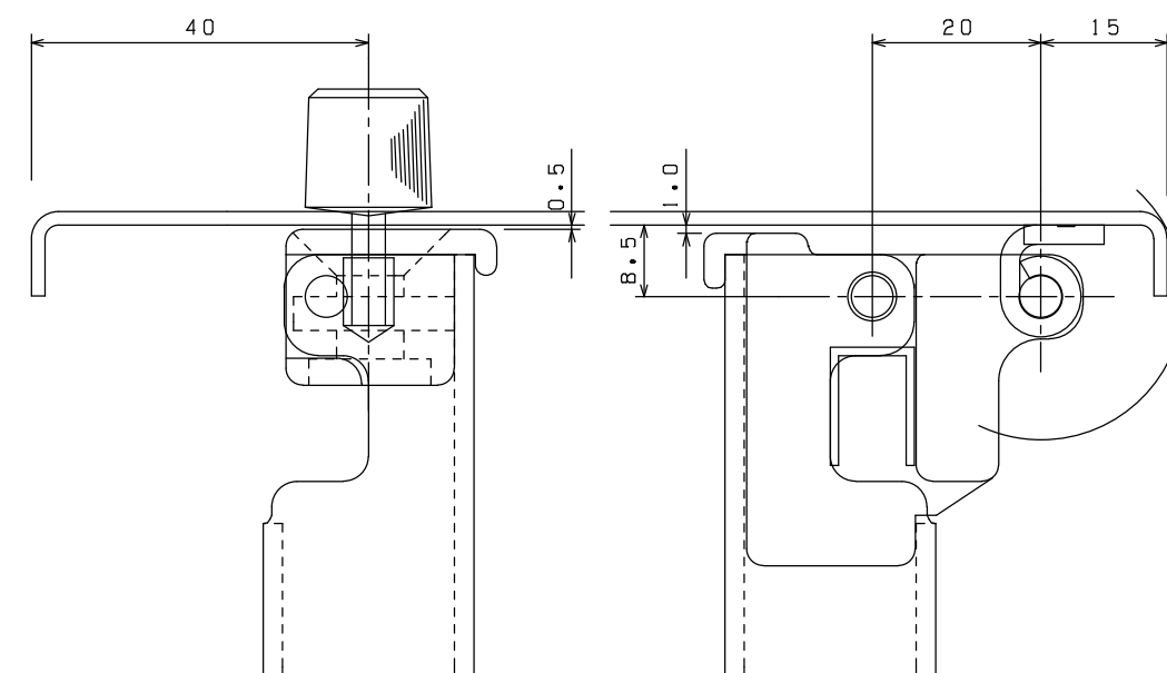
組付け図
